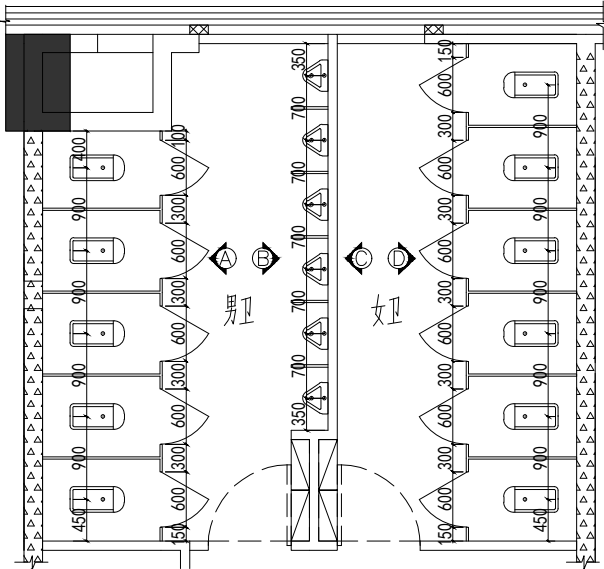
卫生间平面图
