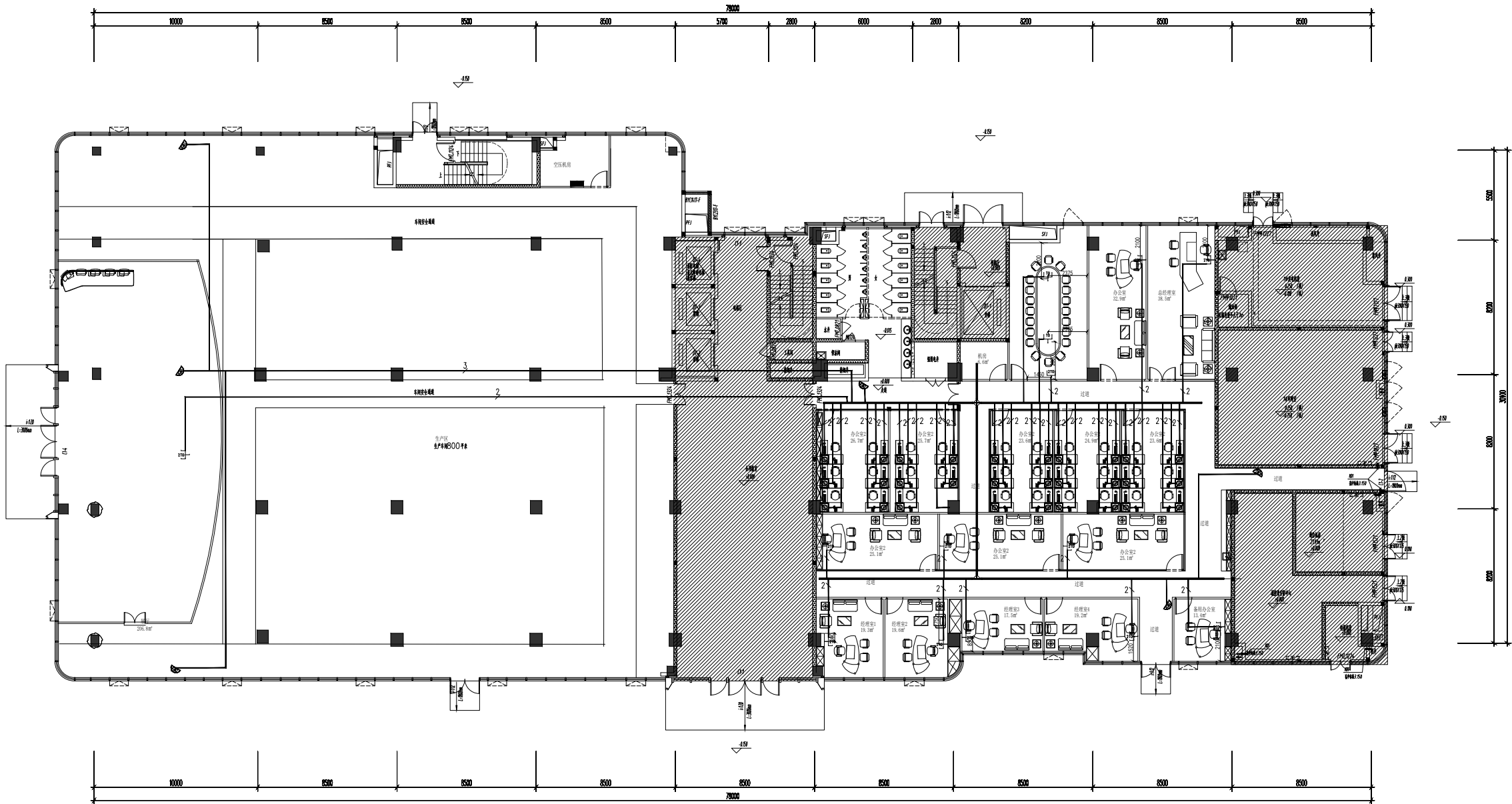
弱电布置图 1:100
