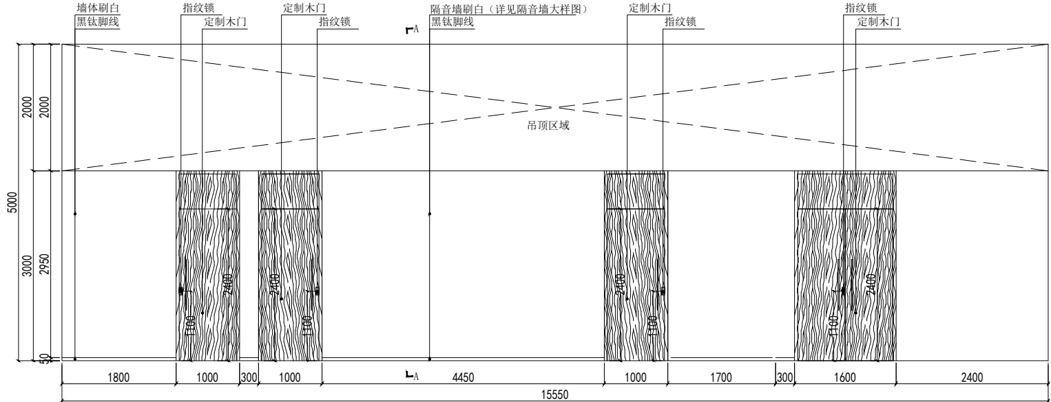
立面图
