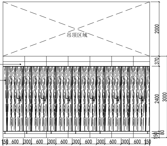
女卫D立面图
