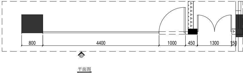
平面图
