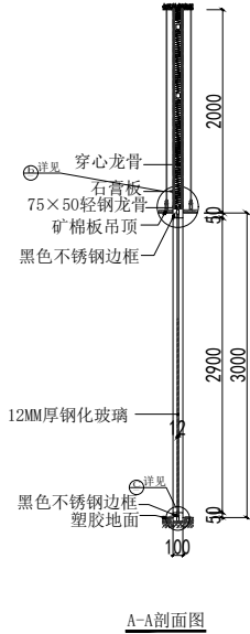
A-A剖面图
