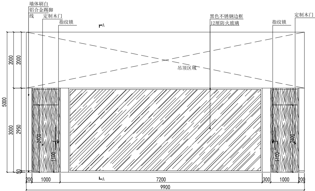
立面图
