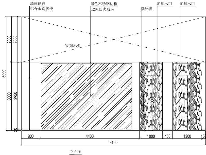
立面图
