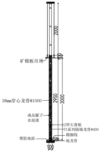
A-A剖面图
