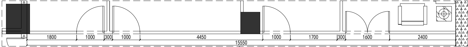
平面图
