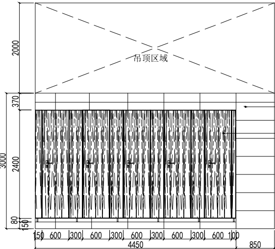
男卫A立面图
