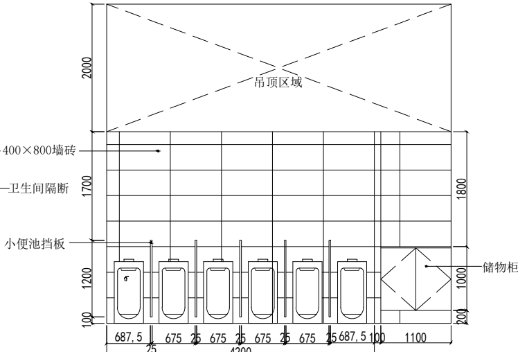
男卫B立面图
