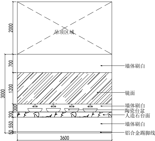
洗手区立面图
